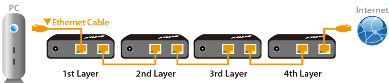
网络界面扩充盒菊花链拓扑类型 1
